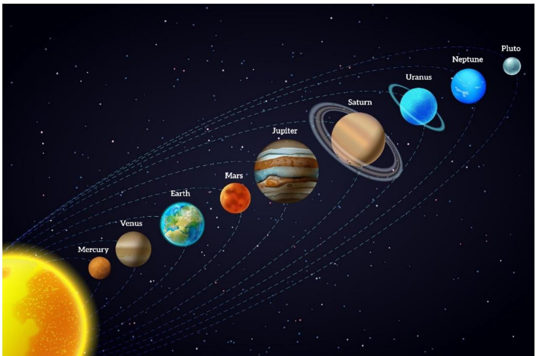
Figuur 1 Ons Zonnestelsel met 9 planeten
