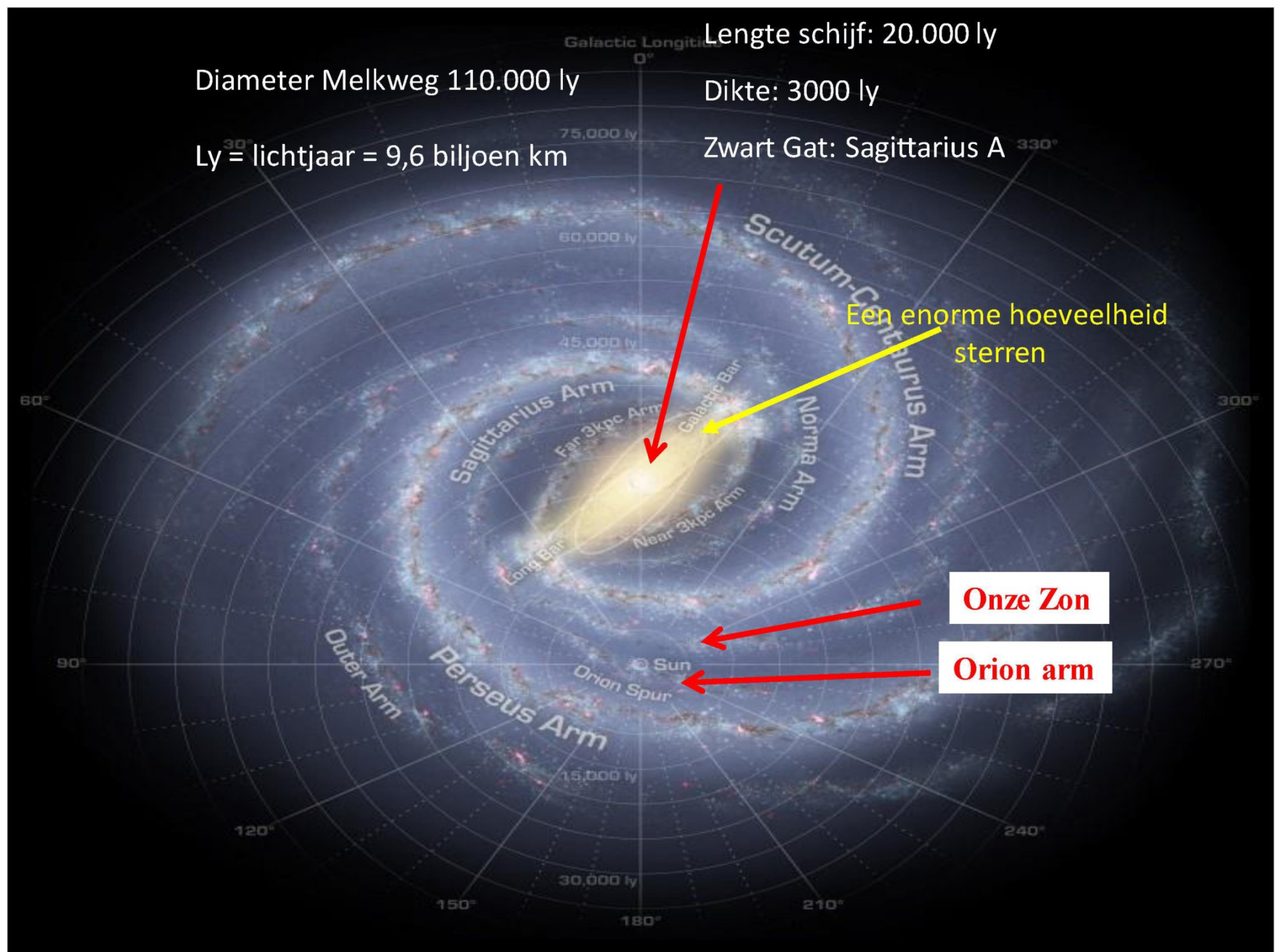
Figuur 3 Onze Melkweg
