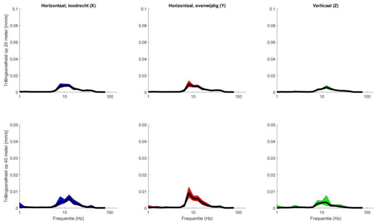
Figuur 45: Trillingspectra (95 procentinterval) op 20 (boven) en 50 (onder) meter afstand
